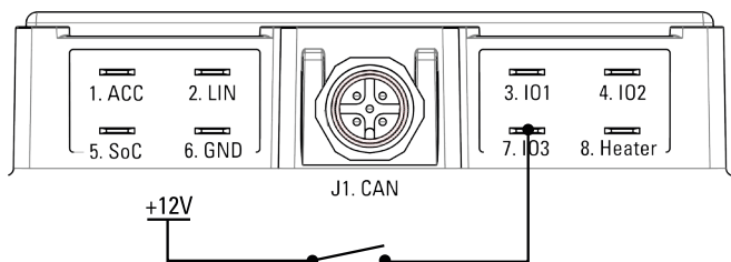
Abbildung 19. Hauptschalter an externe Quelle anschließen
