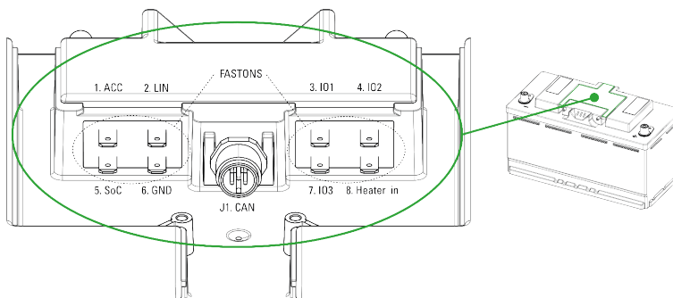
Abbildung 4. Signalschnittstellen
