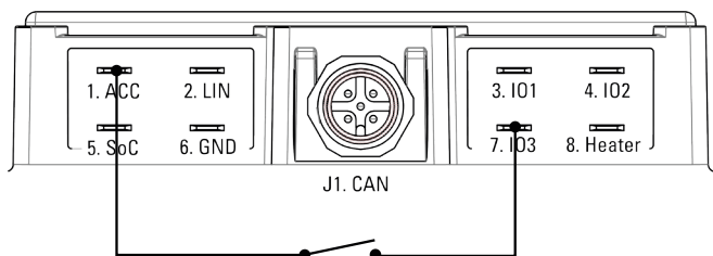
Abbildung 20. Hauptschalter an den Zubehörausgang anschließen
