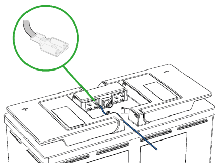
Abbildung 16. Anschluss der LIN-Schnittstelle über den FASTON-Anschluss
