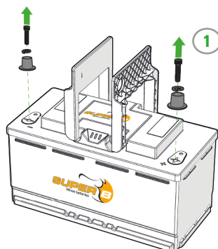
Abbildung 9. Entfernen Sie die Kfz-Batteriepole.
